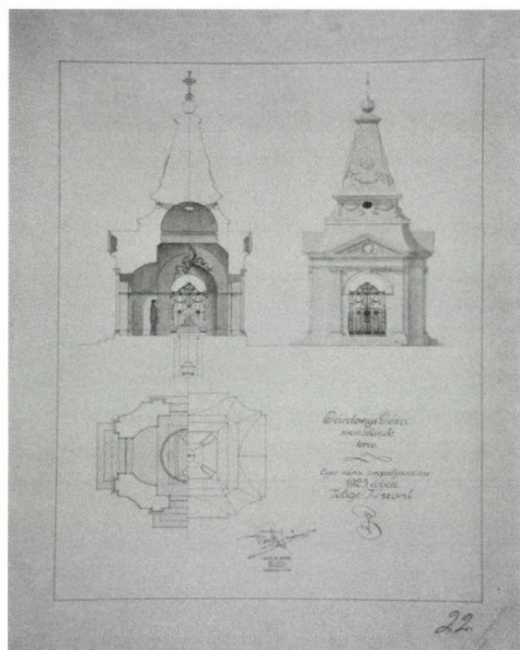
2. a-b kép „Koszori”, Kósch Jenő első helyezett terve
