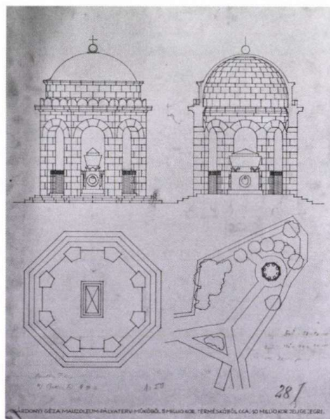
3. kép „Egri”, Müller Tibor első helyezett pályamunkája
